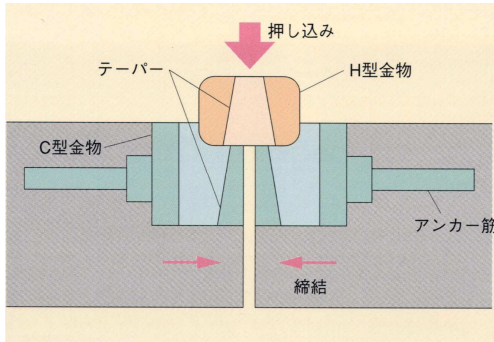
図面-1 地下室接合継手
